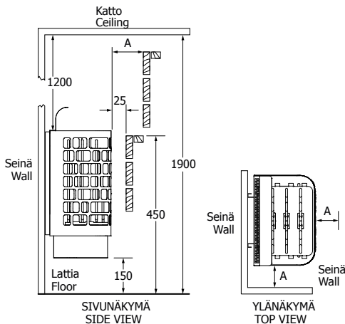
Kuva 1 | Minimisuojaetäisyydet (mm) Fig. 1 | Minimum safety distances (mm)
